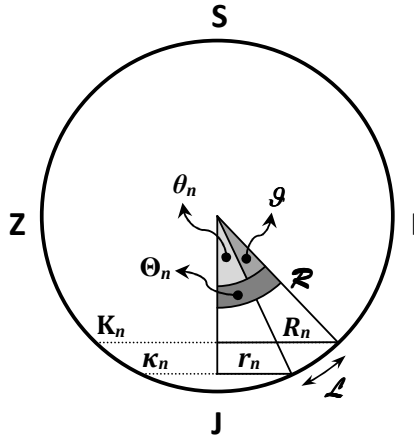
Slika 4: Geometrijske veličine potrebne za analizu problema.
