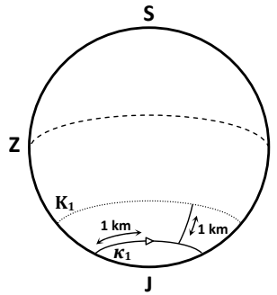
Slika 2: Konstrukcija kružnice K_1 , kao dodatnog rješenja problema.
