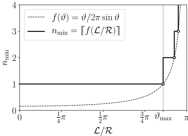
Slika 5: Oblik funkcije (19), kojom je definiran indeks n_{\min} prve kružnice \kappa_n koju je moguće konstruirati u skladu s uvjetima početnog problema.
