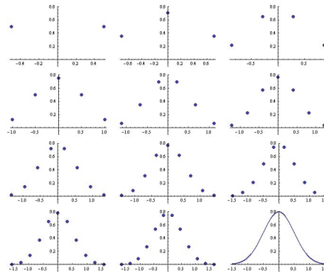
Slika 3. Normalna distribucija kao limes binomnih. Na slikama su za n = 1, \dots, 11 ucrtane točke \left(\frac{k-\frac{n}{2}}{\sqrt{n}}, \frac{\sqrt{n}}{2^n} \binom{n}{k}\right) . Zadnji graf je graf funkcije f(x) = \sqrt{\frac{2}{\pi}} e^{-2x^2} .
