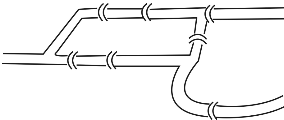
Slika 2. Problem mostova u Königsbergu.
