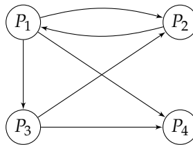
Slika 1: digraf D predstavlja poveznice web stranica
